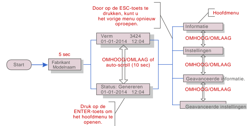
▲ Figuur 6.1 Overzicht bediening
